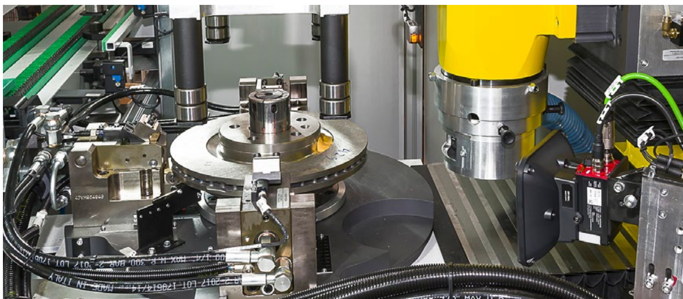
Impianto di equilibratura completo di lettore codice Datamatrix posizionato automaticamente tramite attuatore pneumatico. Balancing system equipped with Datamatrix reader automatically positioned by a pneumatic actuator.
