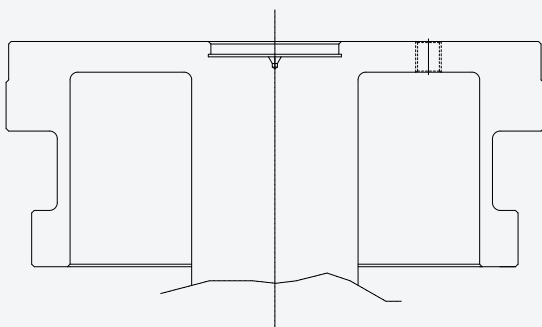
TERMINALE ALBERO NORMALE - STANDARD SHAFT END
