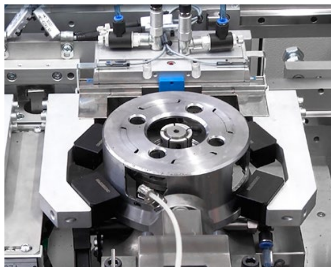
Impianto automatico per la correzione di componenti automobilistici (parti del cambio) con correzione automatica tramite punzonatura orizzontale completa di caricatore lineare e nastri trasportatori.
